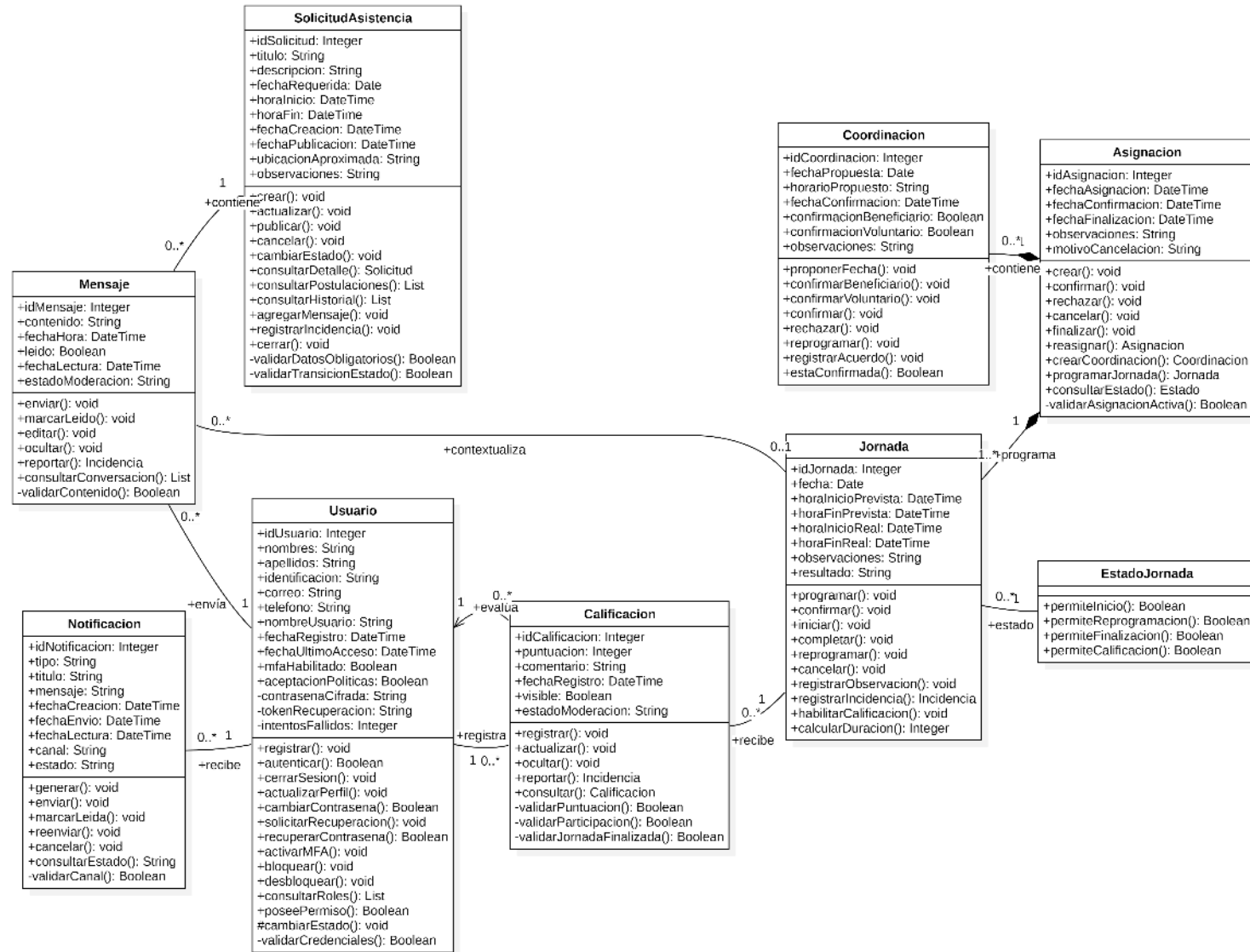
Ilustración 8 Diagrama de coordinación y atención
