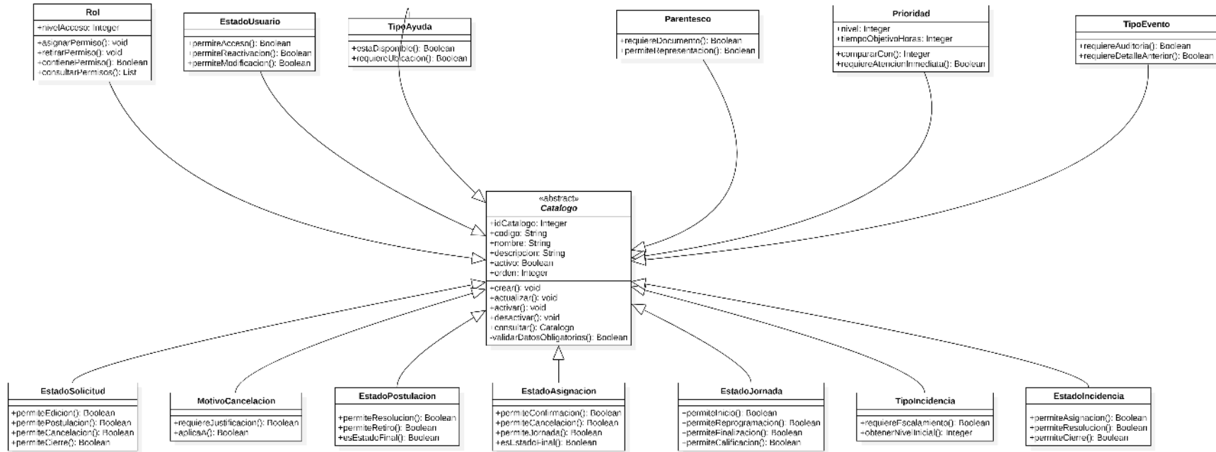
Ilustración 5 Diagrama de catálogos y estados
