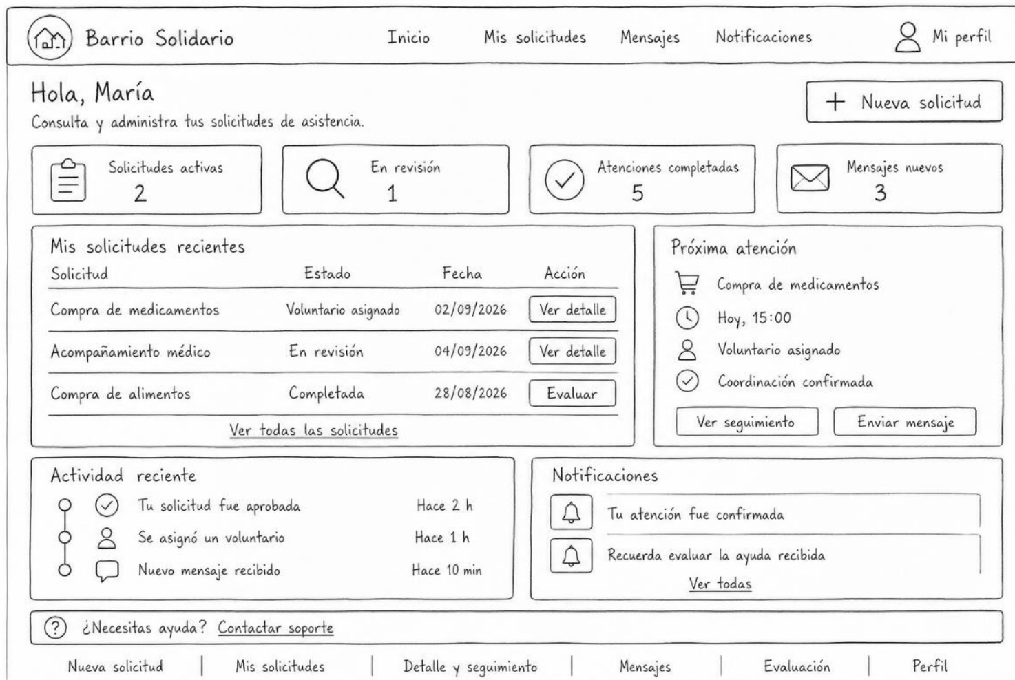
Ilustración 28 Wireframe página panel del solicitante
